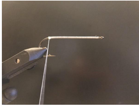
Garnir la hampe avec la soie « bigfly ».
